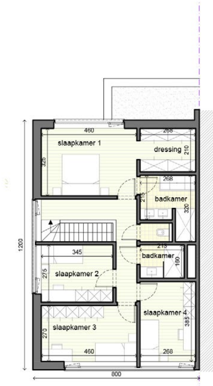
Verdieping
