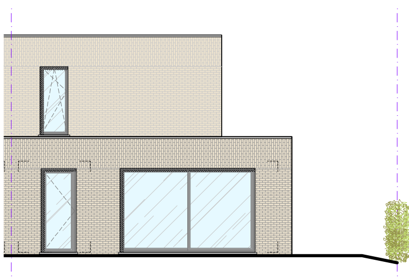
achtergevel
